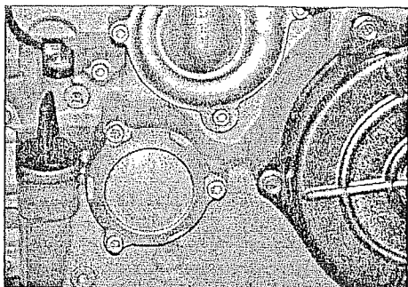
1. Vypouštěcí zátka chladící kapaliny
